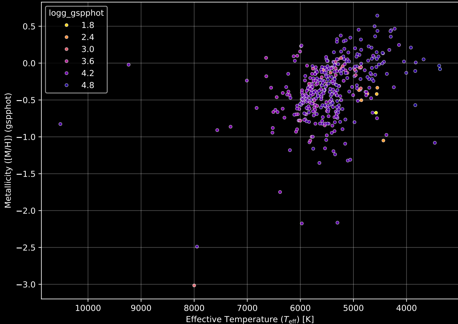
GALAH DR4 Field: [6689] Stellar Population Parameters (n= 407)
