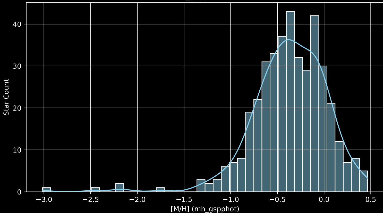
GALAH DR4 Field: [6689] [M/H] (mh_gspphot) (n= 405)
